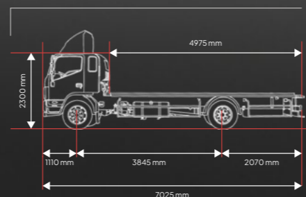
کامیونت ۶ تن خواب دار
