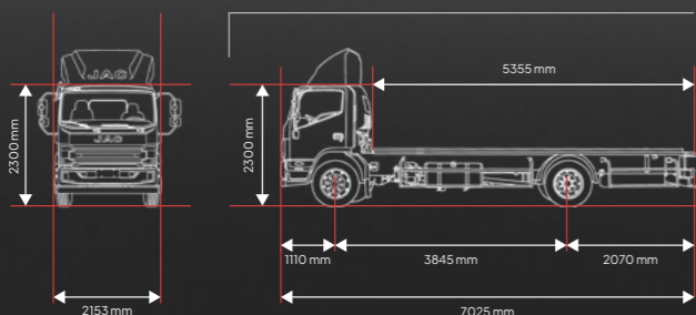
کامیونت ۶ تن بدون خواب
